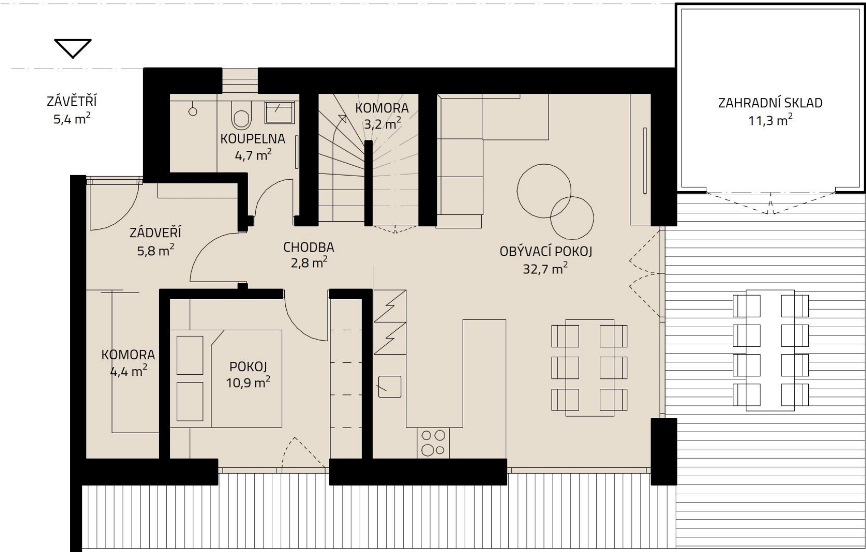
PŮDORYS PŘÍZEMÍ
