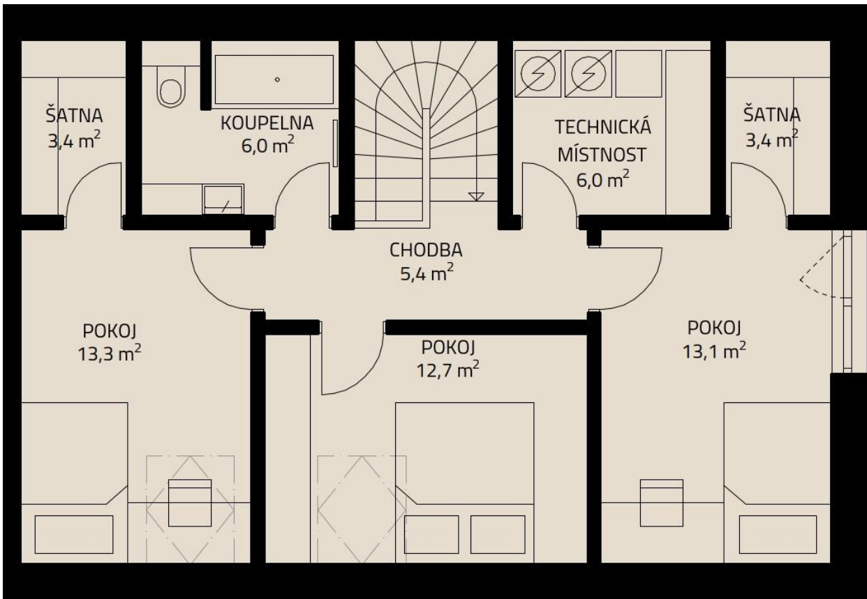
PŮDORYS PODKROVÍ
